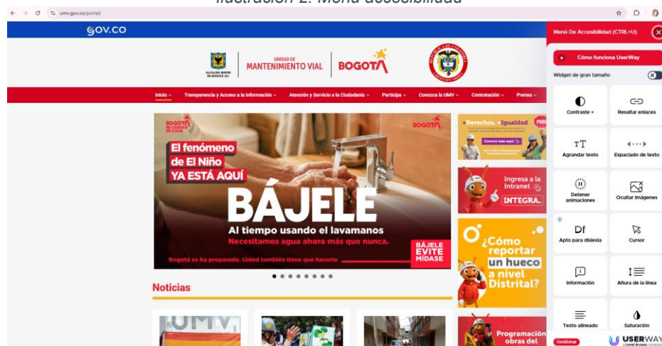
Ilustración 2. Menú accesibilidad
