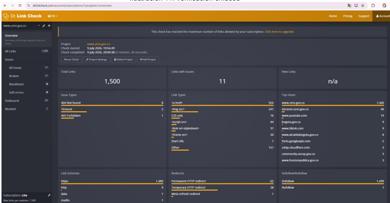
Ilustración 11. verificación enlaces
