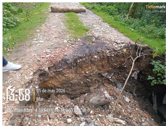
Fotos 6 – 7. Falla en la estructura de soporte o placa de la estructura tipo box coulvert, permitiendo el fallo en el relleno de la vía, materiales de relleno se observa estratos consolidados de escombros con una altura mayor a los 50 cm, no se perciben hombros de la estructura, no se logra identificar estado del descole de la estructura, placa, dentellón, solera, ni aletas.
